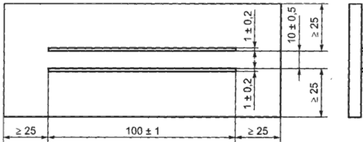
Рисунок 4 - Испытательный образец с электродами из проводящей краски
