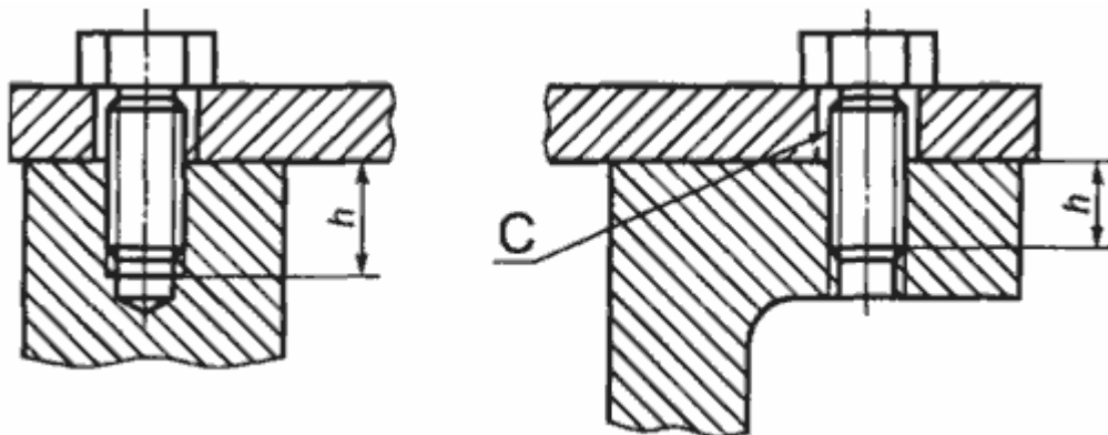
Рисунок 1 - Допуски и зазор для резьбовых крепежных деталей
