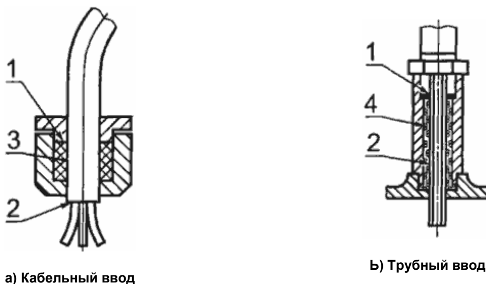
Рисунок 3 - Иллюстрация места ввода корешка и разделки (развода жил) 1 - место ввода кабеля; 2 - место разделки жил кабеля; 3 - уплотнительное кольцо; 4 - герметизирующий компаунд
