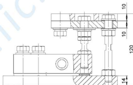
Жорстке кріплення датчика
