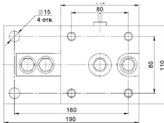
Вільно-оперте кріплення датчика Мінімальне
