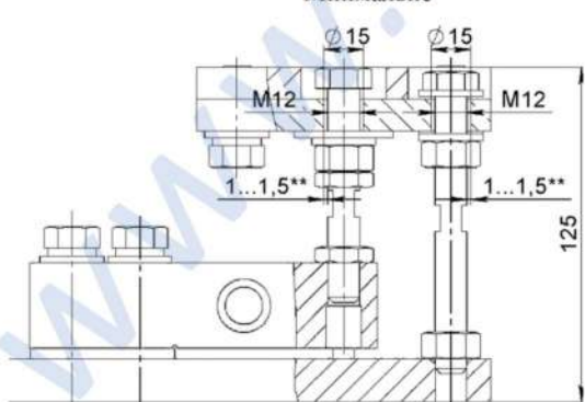
Вільно-оперте кріплення датчика Мінімальне
